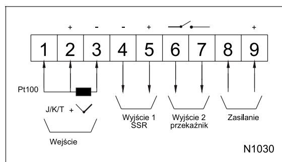
SCHEMAT POŁĄCZEŃ
