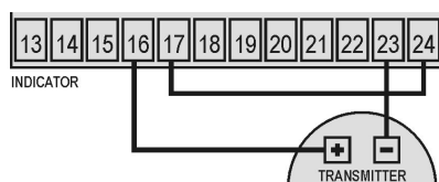
Rys. 9 – Dwu-przewodowy transmiter z wewnętrznym zasilaniem
