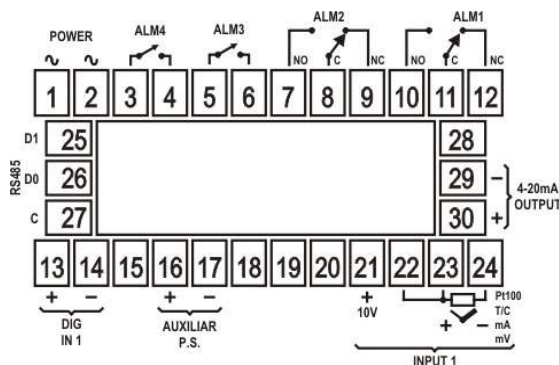
Rys. 2 – Zaciski na panelu z tyłu wskaźnika
