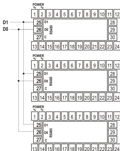
Rys. 11 – Połączenia w sieci RS-485
